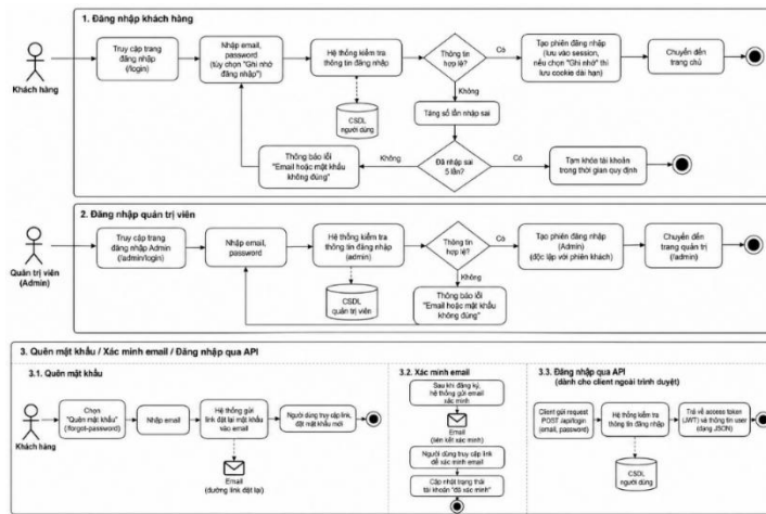
Hình 1.2.1.2 Luồng đăng nhập / xác thực
