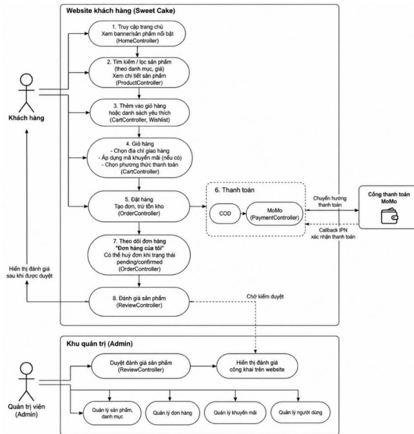
Hình 1.2.1.1 Luồng mua hàng của khách (E2E)
